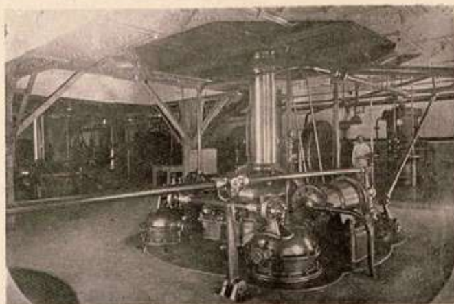
Cilindros reguladores; mancal de eixo; válvula para admissão d'água na turbina de 18.000 H. P.
