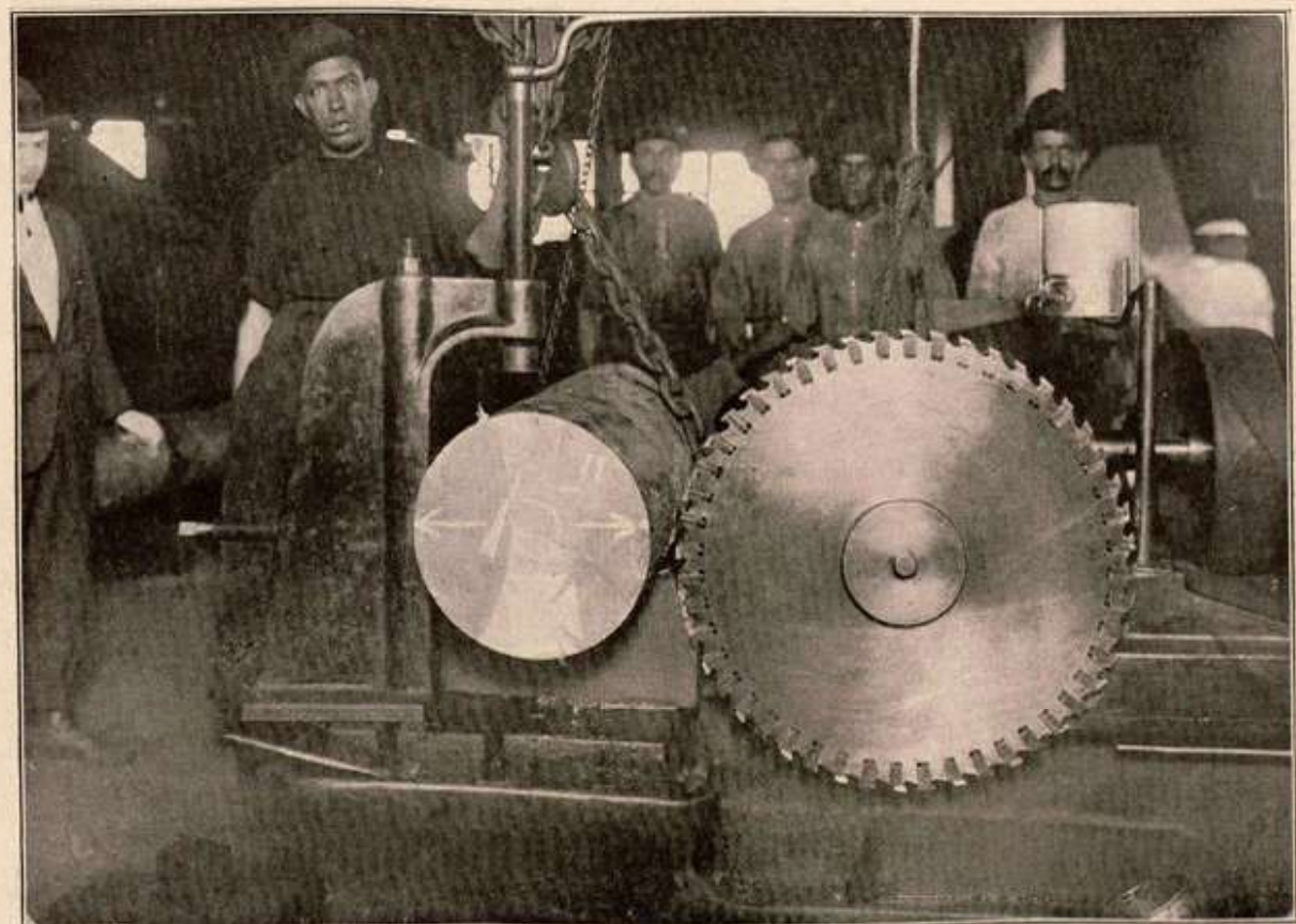
Serra circular para ferro
