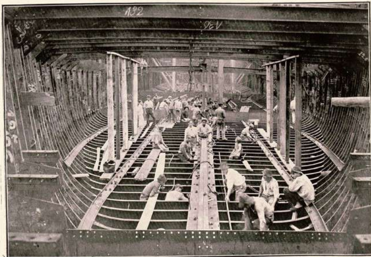
A CONSTRUÇÃO DO "ITAQUATIÁ" NA ILHA DO VIANNA
