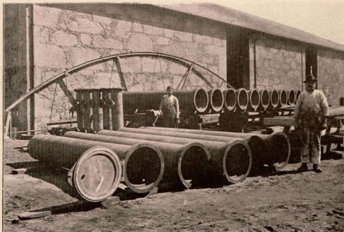
Tubos fundidos na ilha do Vianna — C. N. Navegação Costeira
