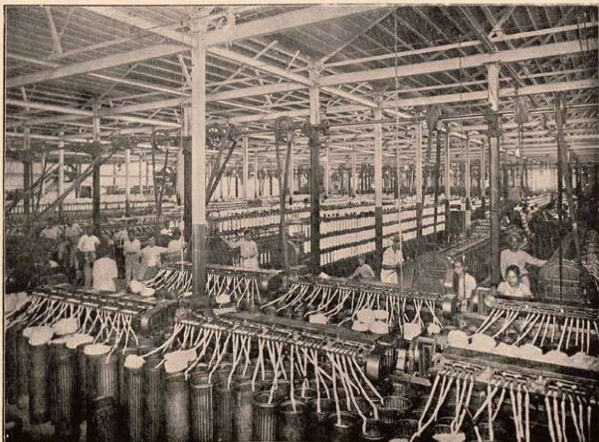
Passadizas—Massarquitira. Fabrica de Tecidos Nossa Senhora da Conceição—Campos
