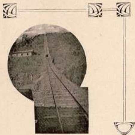
Piano inclinado da usina a 10°
