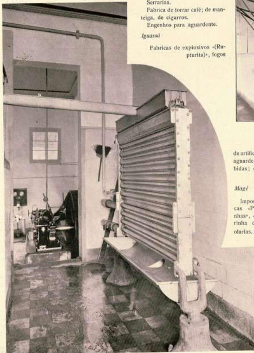
Rebolsamento do leite na Fabrica de Lacticos e Gelo —Barra do Pirahy
