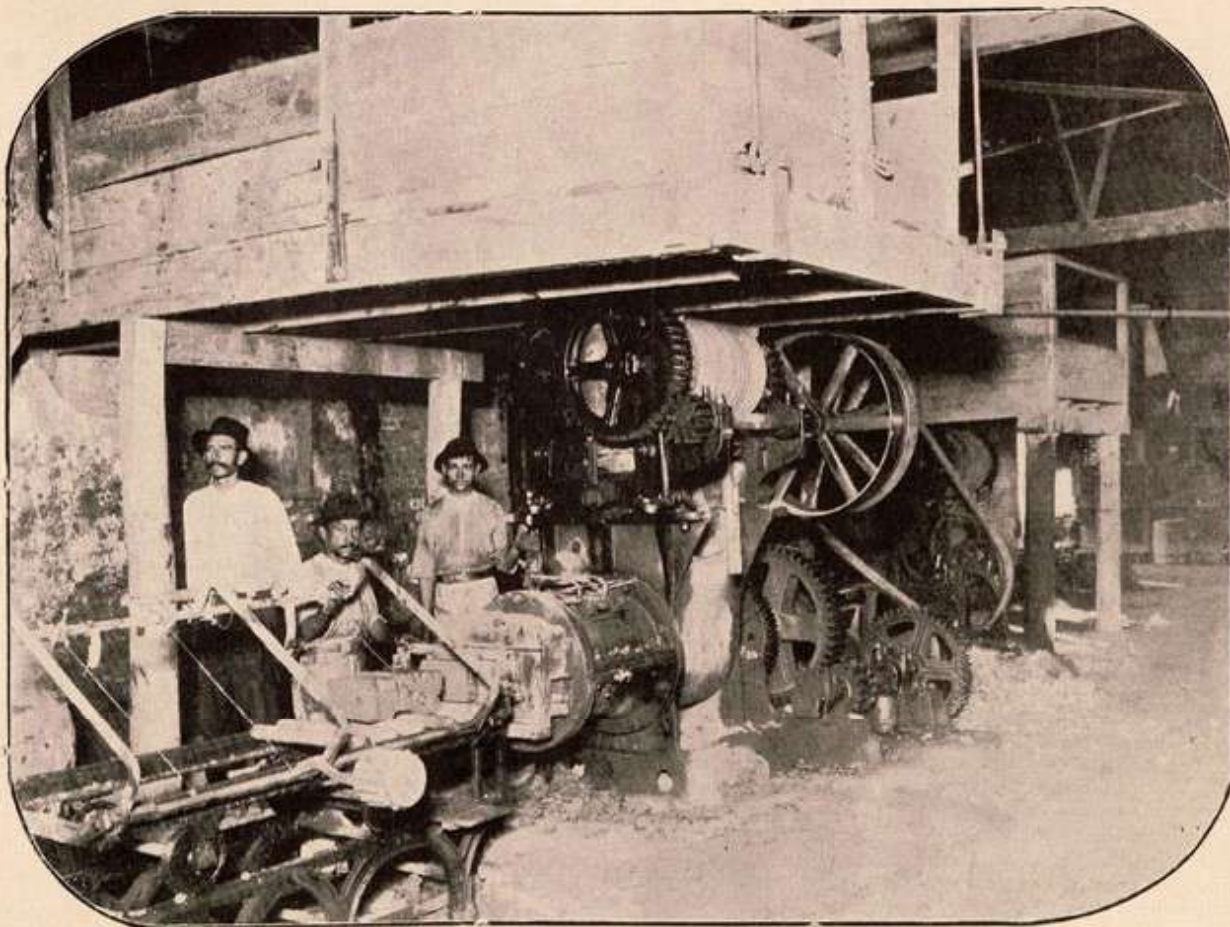
MACHINAS PARA O FABRICO DE TELHAS — PORTO DO ROSA
