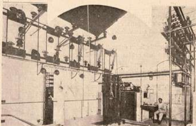
Interior de uma estação de manobra e redução de voltagem
