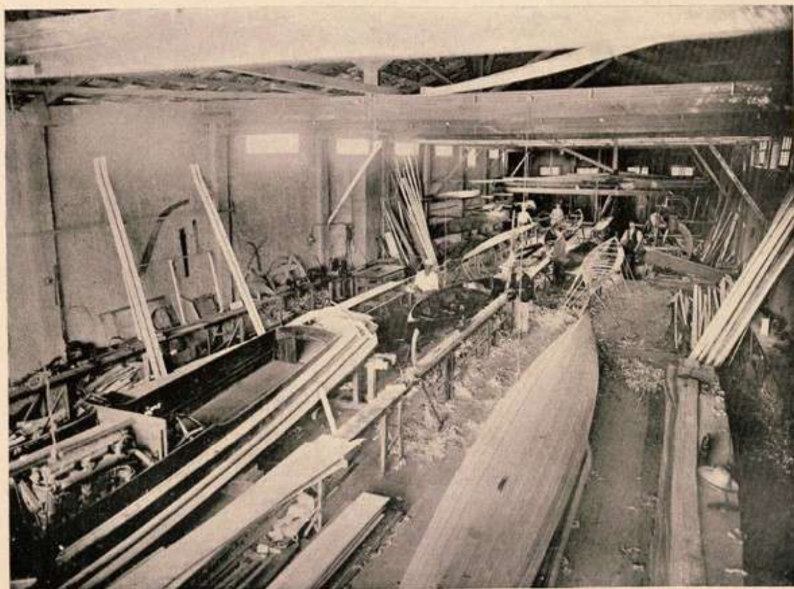
Estalhoiro para construção de embarcações para desporto — Niteróy — Sacco de S. Francisco — M. Jacke
