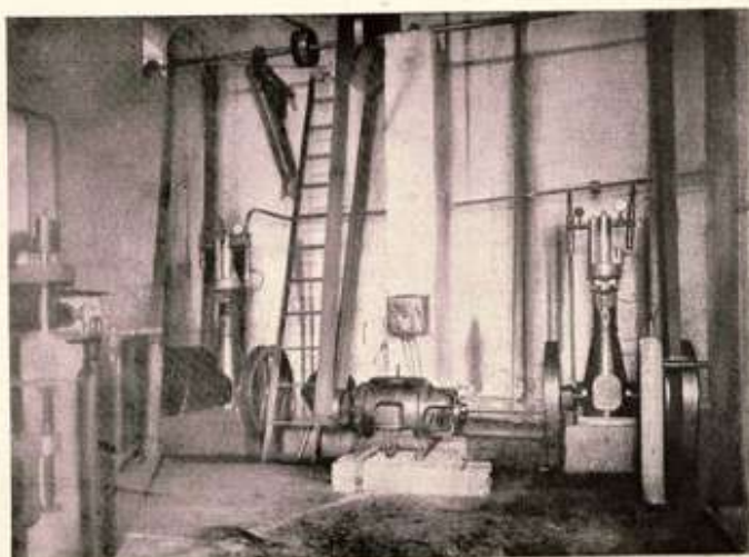
Machina para a congelação do leite
